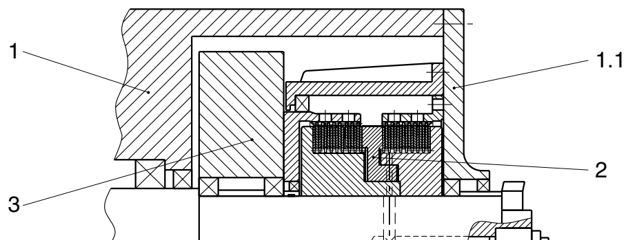
Abb. 4: Einbauvariante 2
