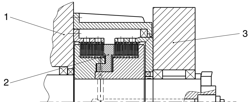
Abb. 3: Einbauvariante 1
