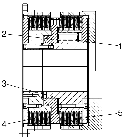
Abb. 1: Funktion der Kupplungs-Bremskombination
